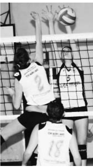
Frassati-Cassini
